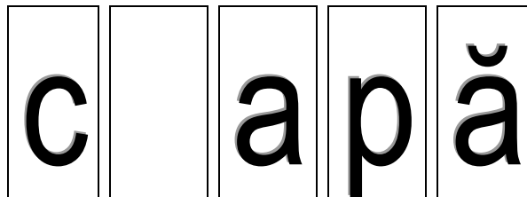
Fig. 3 – literele alfabetului
